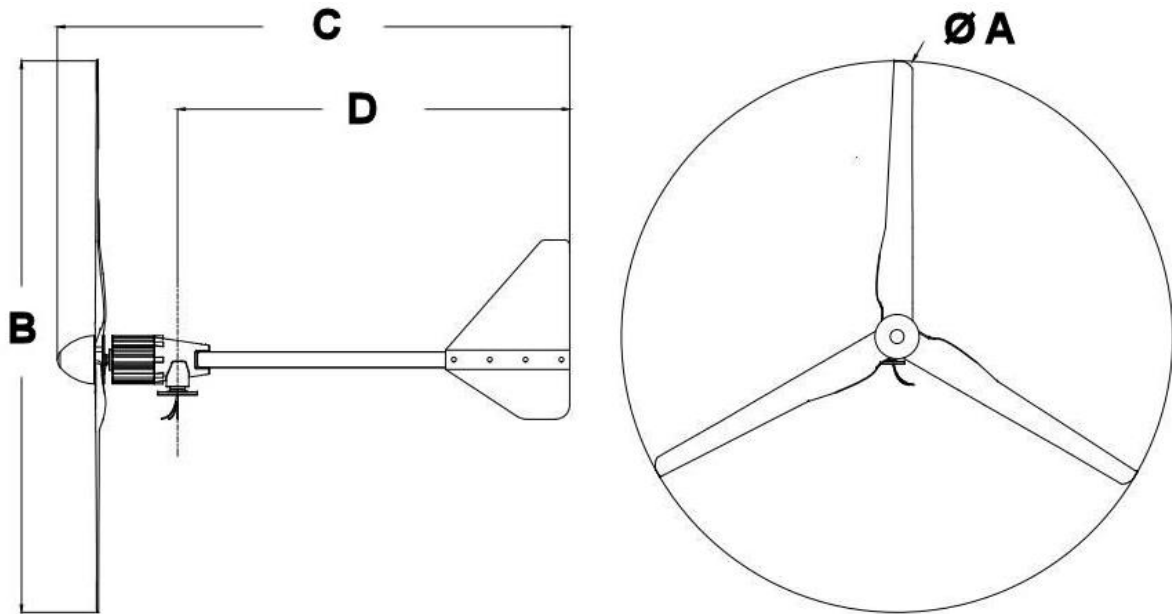
Dimensiones de Generación Eléctrica: Controladores Eólico, SpaceKit.
