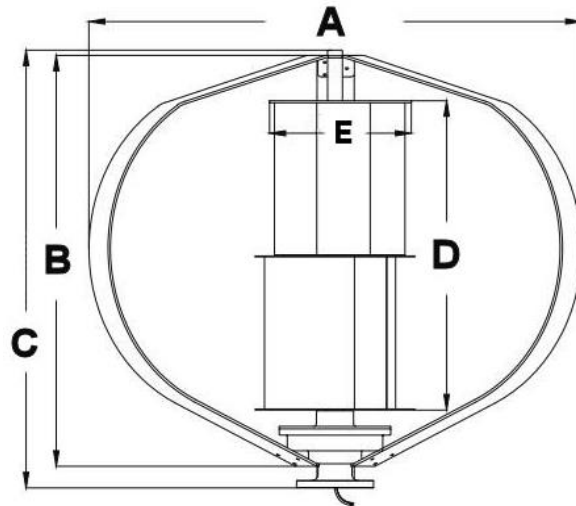
Dimensiones de Generación Eléctrica: Controladores Eólico, GoodKit.
