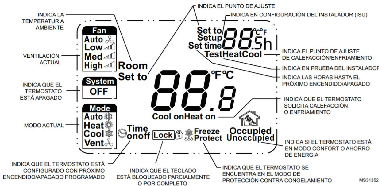
Fig. 2. Pantalla LCD.
