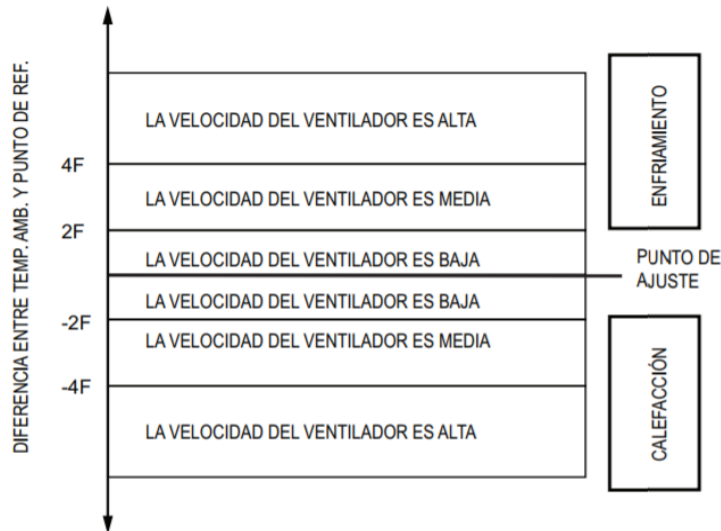
Algoritmo de control del cambio de velocidad del ventilador
