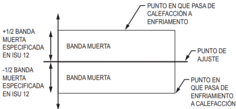
Algoritmo para cuatro tubos con cambio automático y un solo punto de ajuste.
