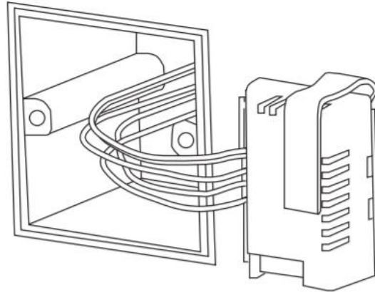
Colocación de los cables en el bloque de terminales.
