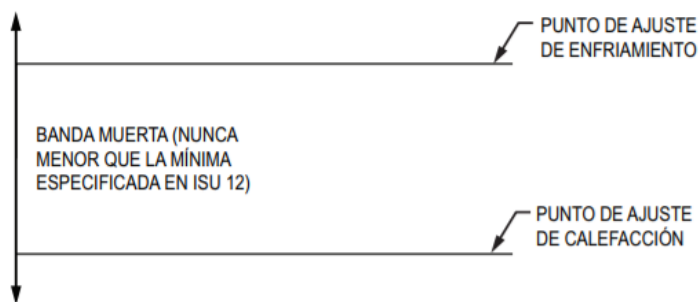
Algoritmo para cuatro tubos con cambio automático y dos puntos de ajuste.
