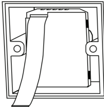
Montaje del módulo de alimentación
