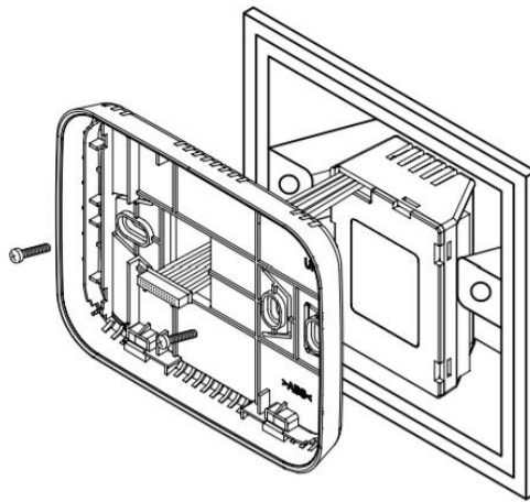
Montaje de la base posterior
