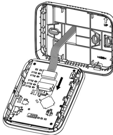
Conexión del termostato
