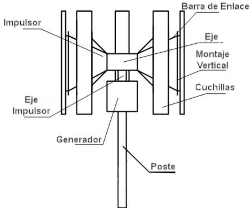
Diagrama de Generación Eléctrica: Generador Eólico Vertical, TwisterKit.
