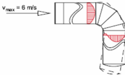
Codo de 90°
