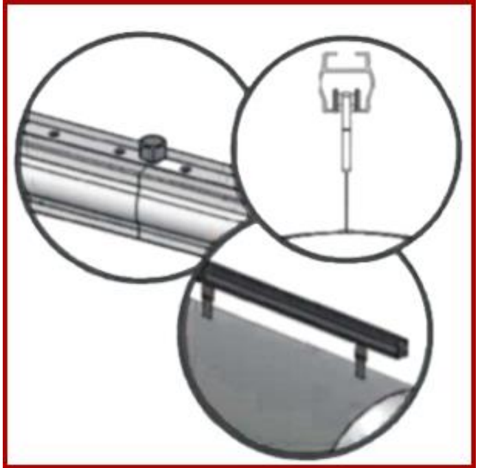
Sistema de Rieles para Ducto
