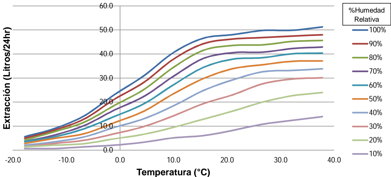
Curva de Extracción de Agua DD400 (Litros/día)
