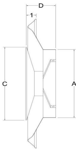
CORTE X-X
