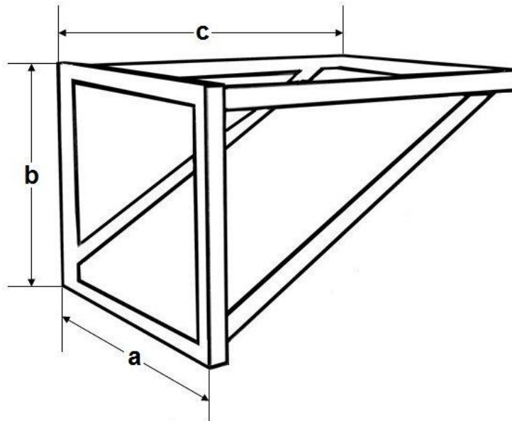
Dimensiones (mm)
